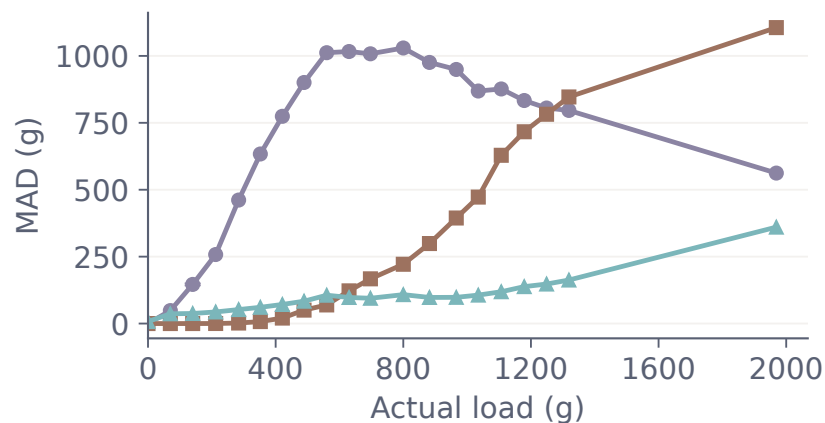
(d) Median absolute deviation
